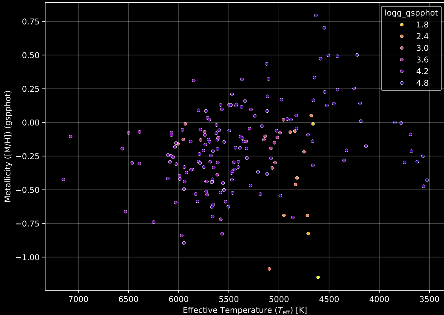
APOGEE DR17 Field: [JHelium6] Stellar Population Parameters (n= 184)
